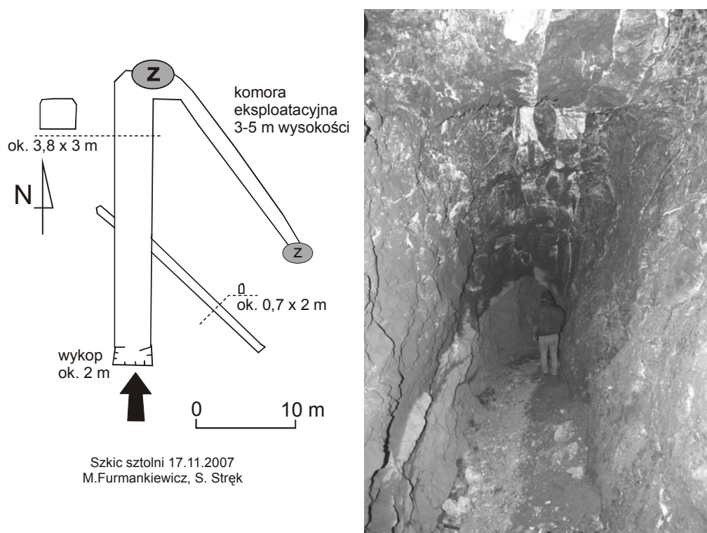
Rys. 5. Schematyczny plan sztolni zachowanej w rejonie kopalni „Grochów 1” (po lewej), oraz widok komory eksploatacyjnej (po prawej, fot. M. Furmankiewicz). Symbol ② oznacza zawał
